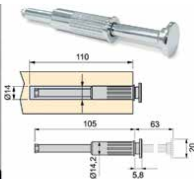
Uitschuifbare kledinghaak
